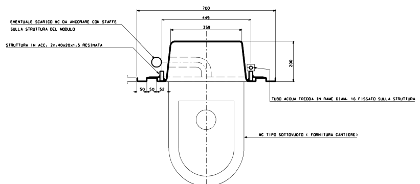
PIANTA
